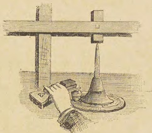
Fig. 35. — Meule de polissage.
